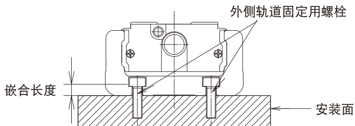
图 4 SKR/KR 安装图
